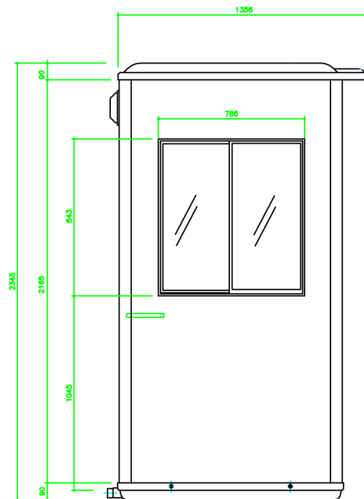
正面図
