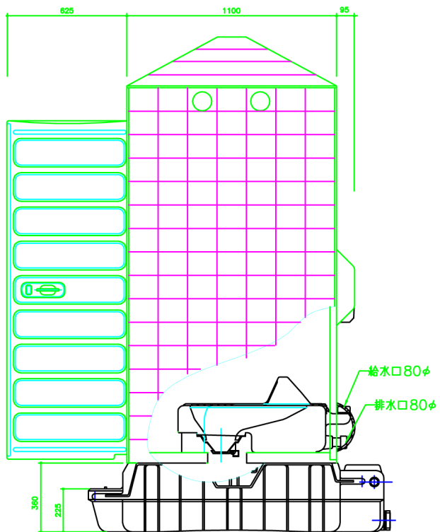
側面図
