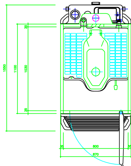
平面図
